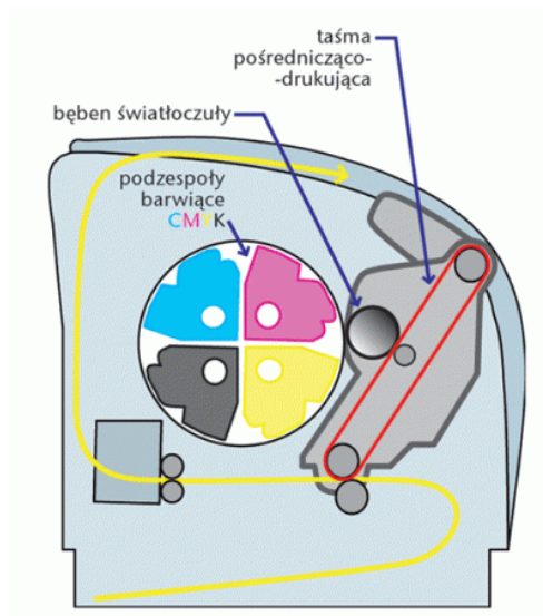
mechanizm druku czteroprzebiegowego
