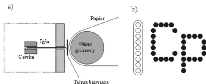
Schemat budowy drukarki igłowej
