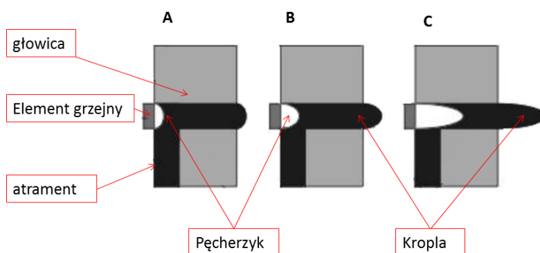
Schemat powstawania kropli w głowicy drukarki atramentowej
