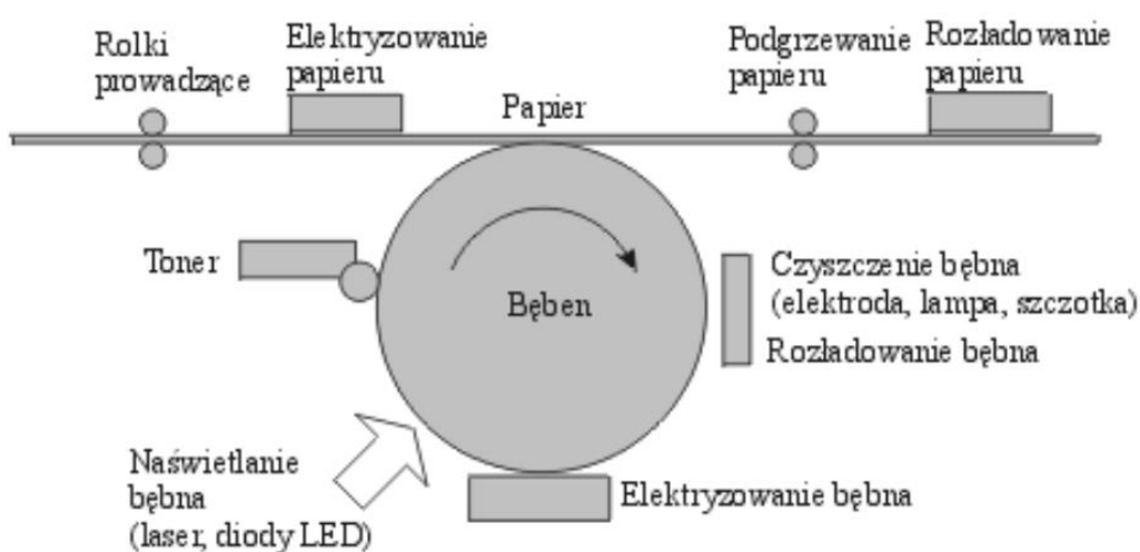
Schemat powstawania wydruku w drukarce laserowej
