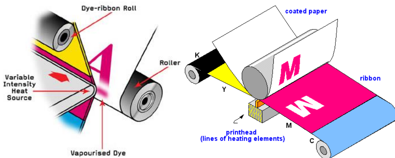
Zasada działania drukarki termosublimacyjnej
